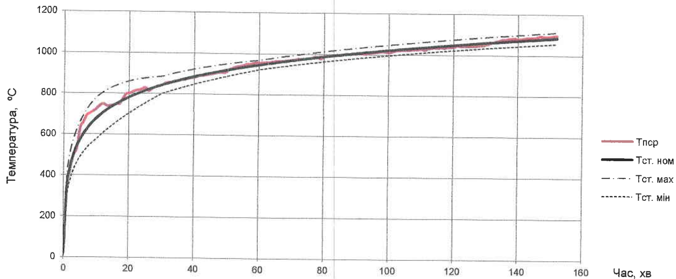
Рис. 3 Температура в печі (зразок №1)
