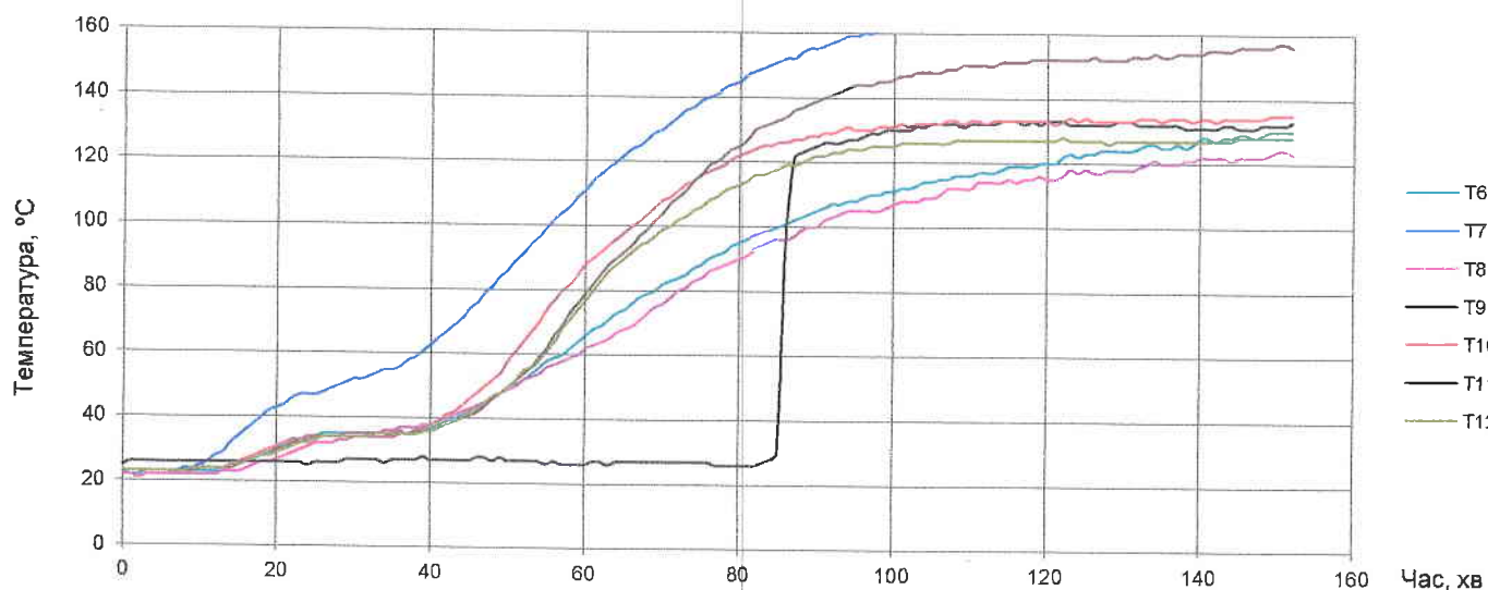
Рис. 5 Температура необігріваної поверхні зразка №1 (T6-T12)
