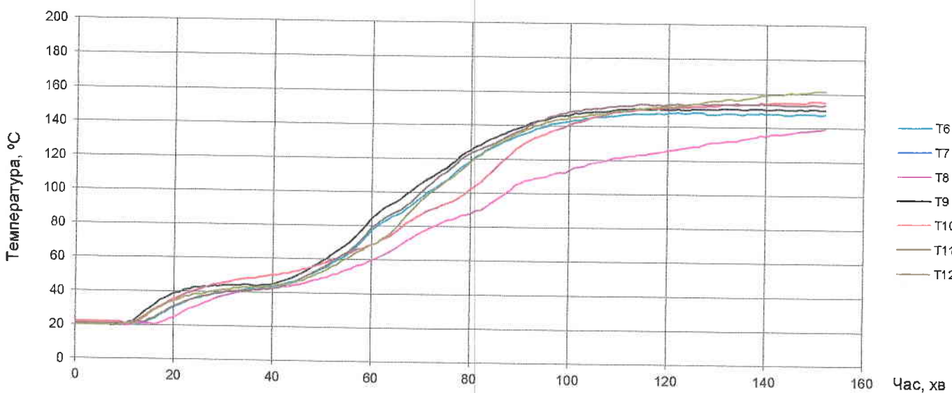
Рис. 8 Температура необігріваної поверхні зразка №2 (T6-T12)
