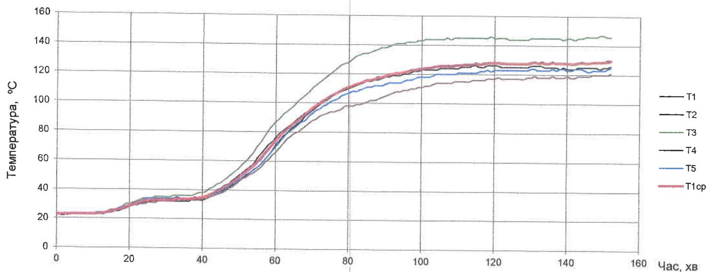
Рис. 4 Температура необігріваної поверхні зразка №1 (T1-T5) та середня температура (T1ср)
