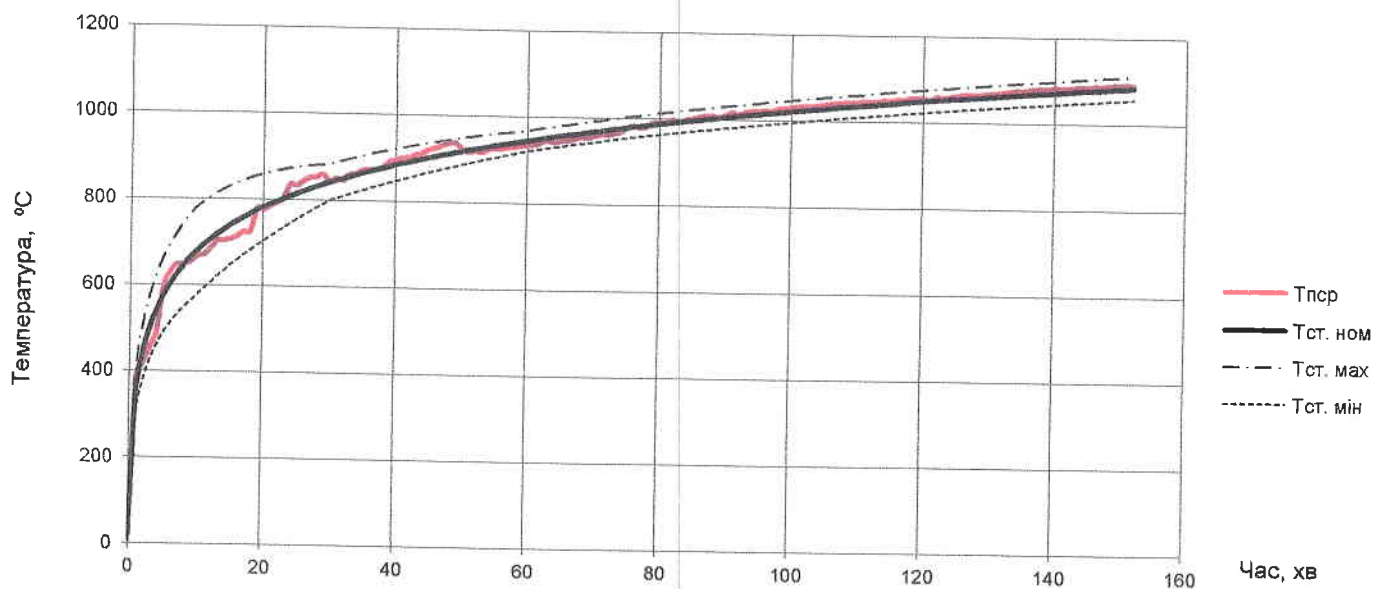
Рис. 6 Темпетатура в печі (зразок №2)
