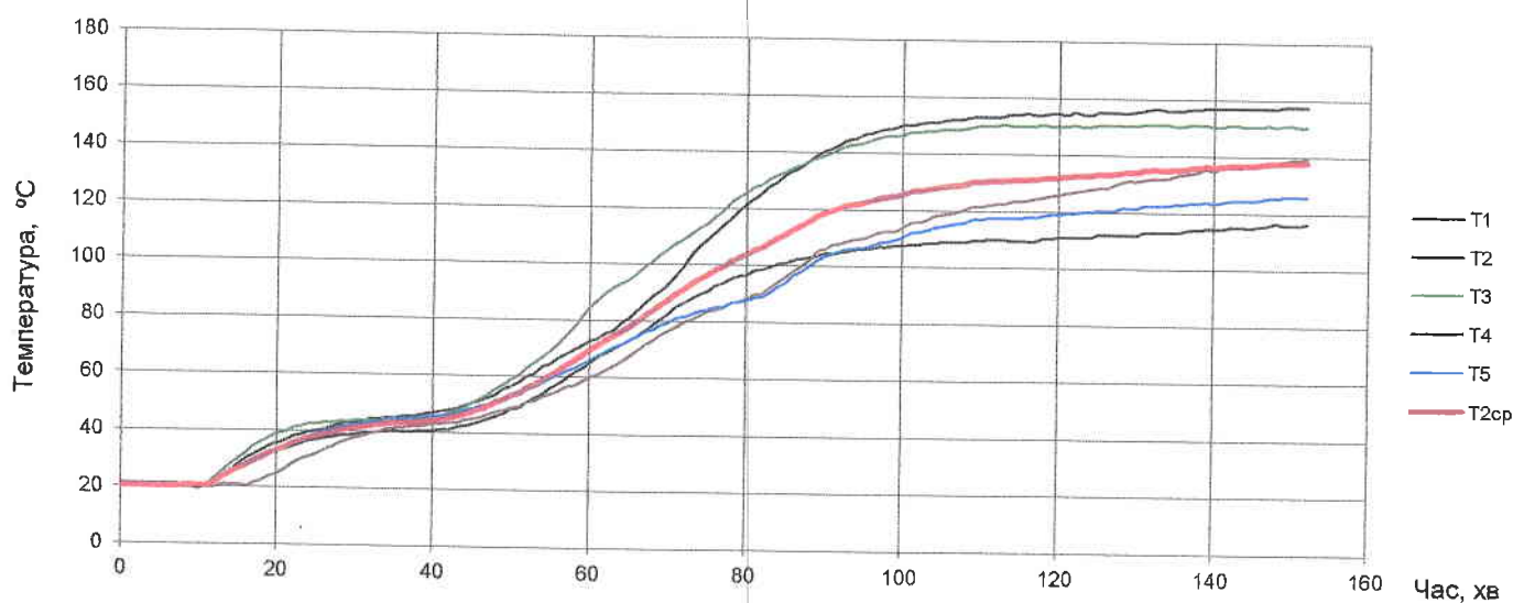
Рис. 7 Температура необігріваної поверхні зразка №2 (T1-T5) та середня температура (T2cp)
